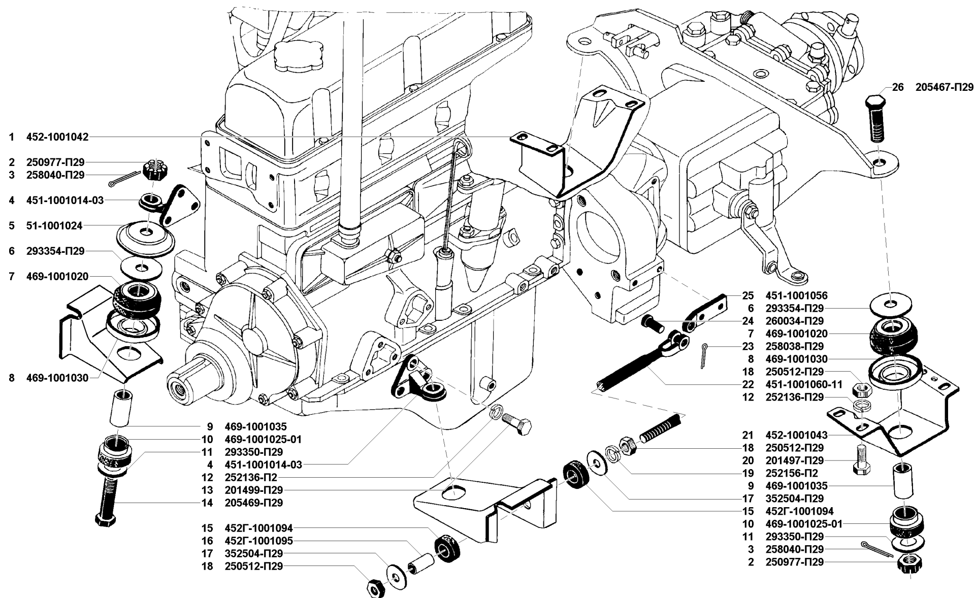
Рис. 2. Подвеска двигателя (1001)
